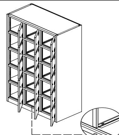
5 Монтирайте горните разделители от ляво на дясно.
