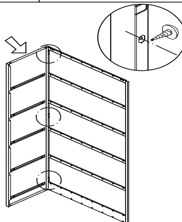
1 Захванете лявата част към гръба с помощта на винтовете.
