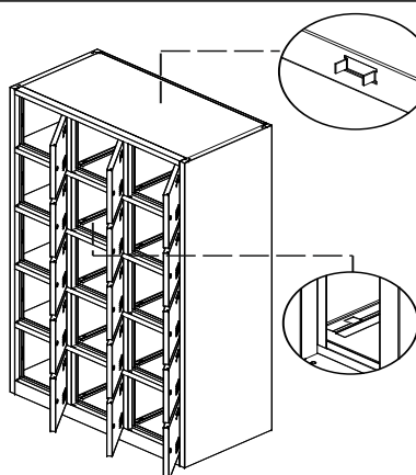
4 Поставете капака, средата и дъното едно след друго.
