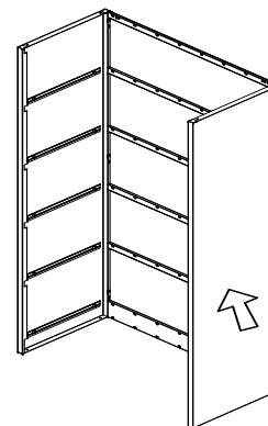
2 Добавете дясната част към гръба по същия начин като на стъпка 1.
